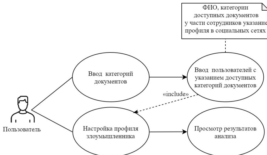
Рис. 3. Диаграмма использования
